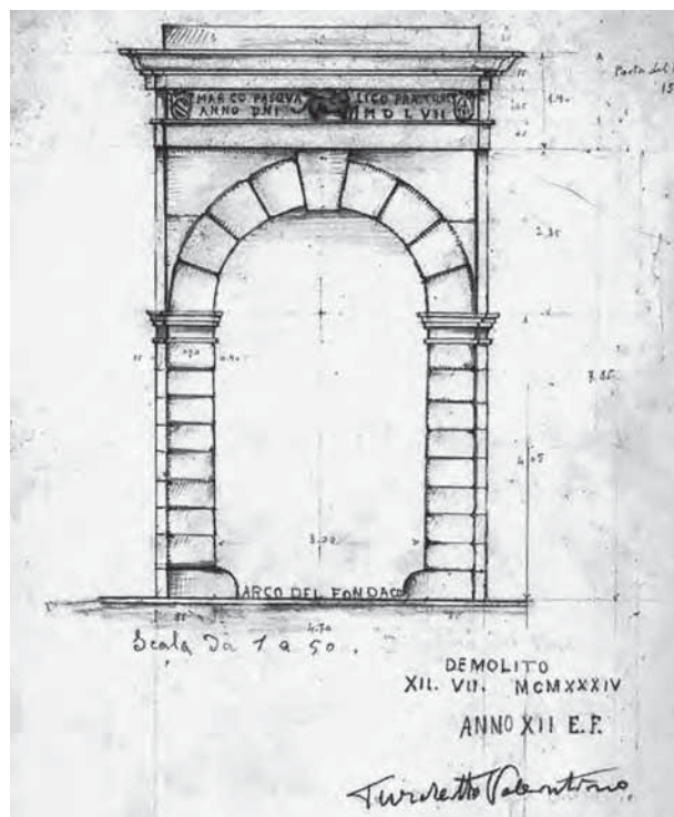
Valentino Turchetto, disegno dell’Arco del Fondaco, 1934 (Archivio Storico Comune di Portogruaro, b. 1590)
